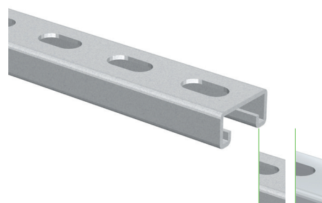
Ankerskinne, kraftig (41x41)
