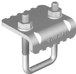
41x21 mm klemme, I-jern
